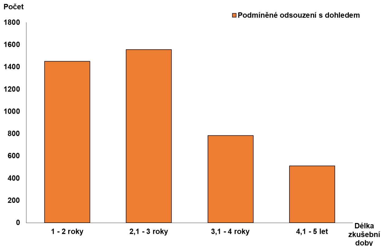
Graf 19 – Délka zkušební doby u podmíněně odsouzených v roce 2021
