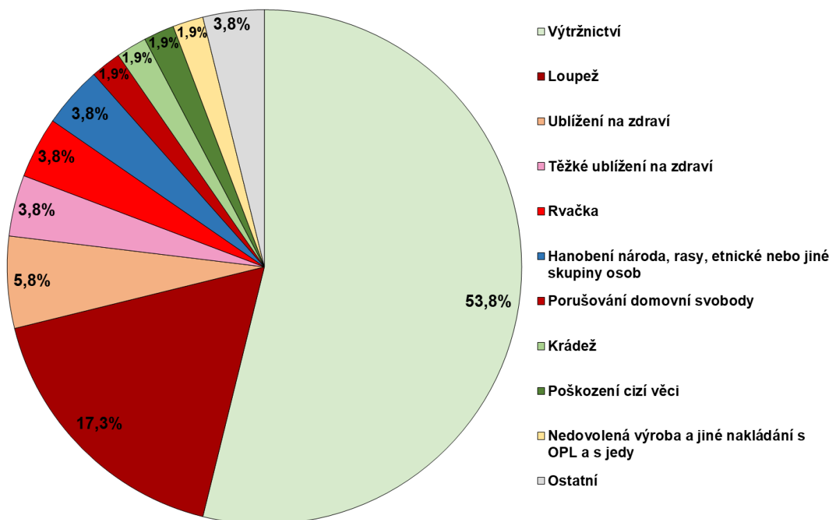
Graf 36 – Struktura trestné činnosti u trestů zákazu vstupu za rok 2021
