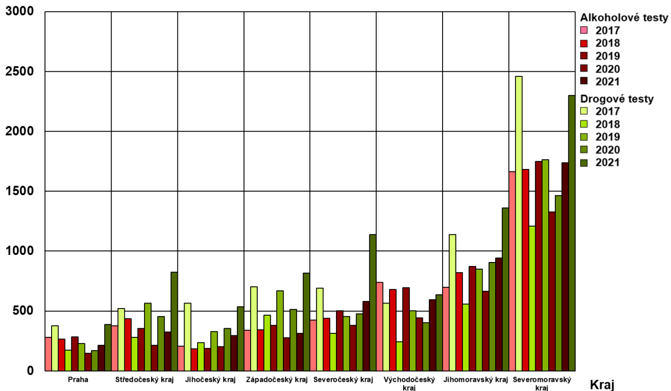
Graf 40 – Počet provedených testů v rámci soudních krajů
