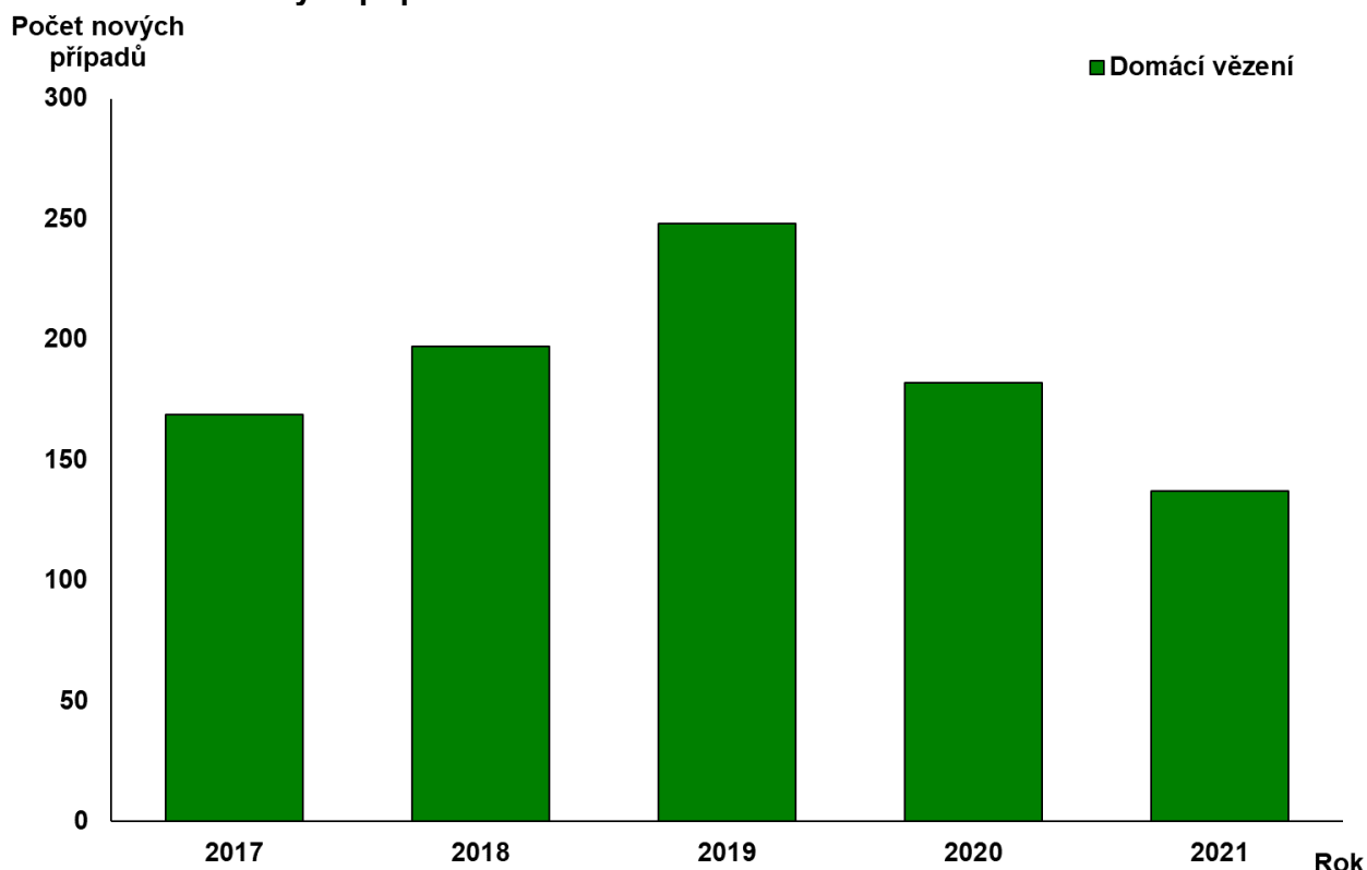
Graf 28 – Počet nových případů domácího vězení
