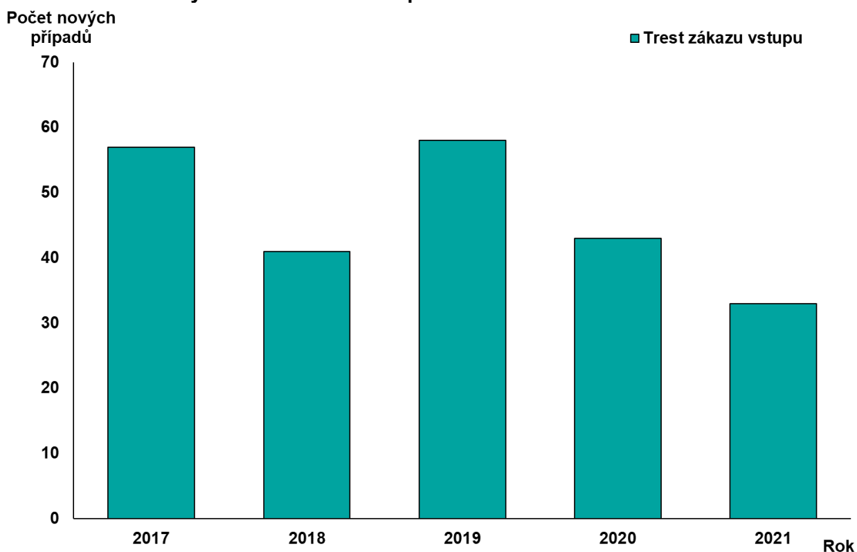
Graf 33 – Počet nových trestů zákazu vstupu
