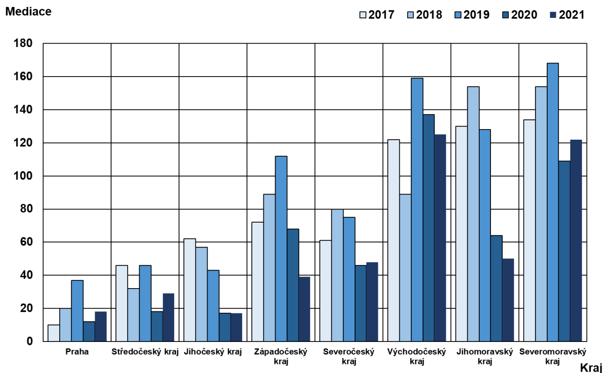
Graf 11 – Počet mediací v rámci soudních krajů
