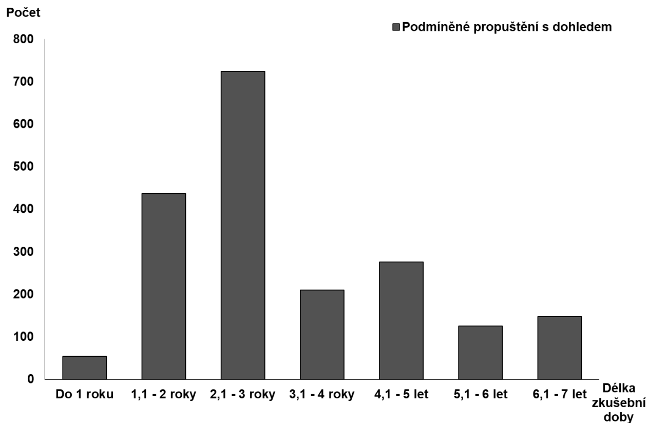
Graf 20 – Délka zkušební doby u podmíněně propuštěných v roce 2021
