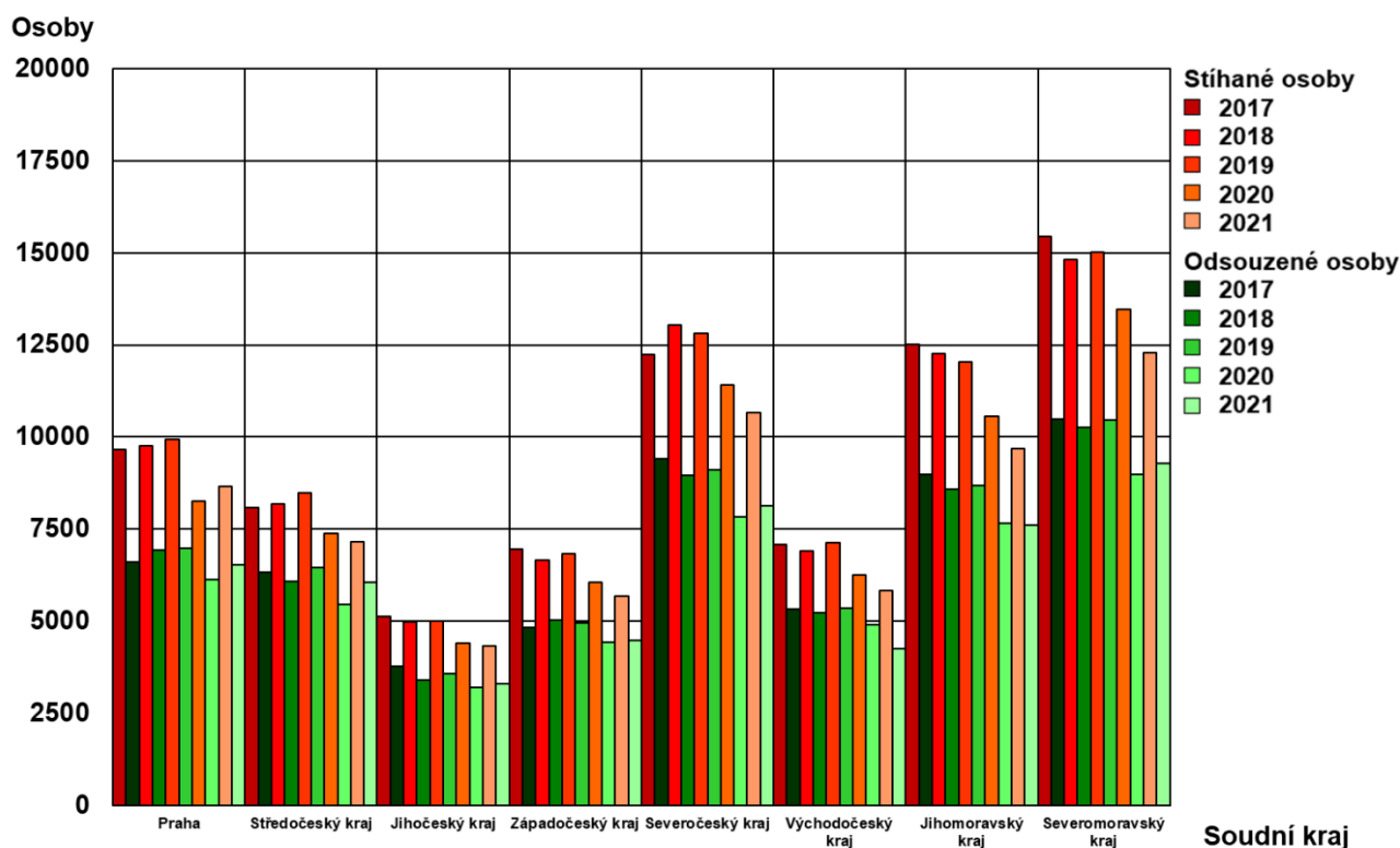
Graf 2 – Vývoj počtu stíhaných a odsouzených osob v soudních krajích 2017–2021
