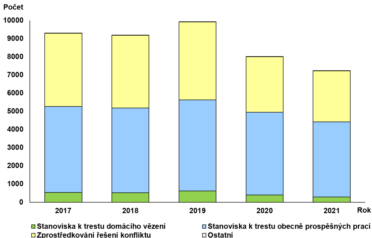
Graf 4 – Počet zpracovaných výstupů
