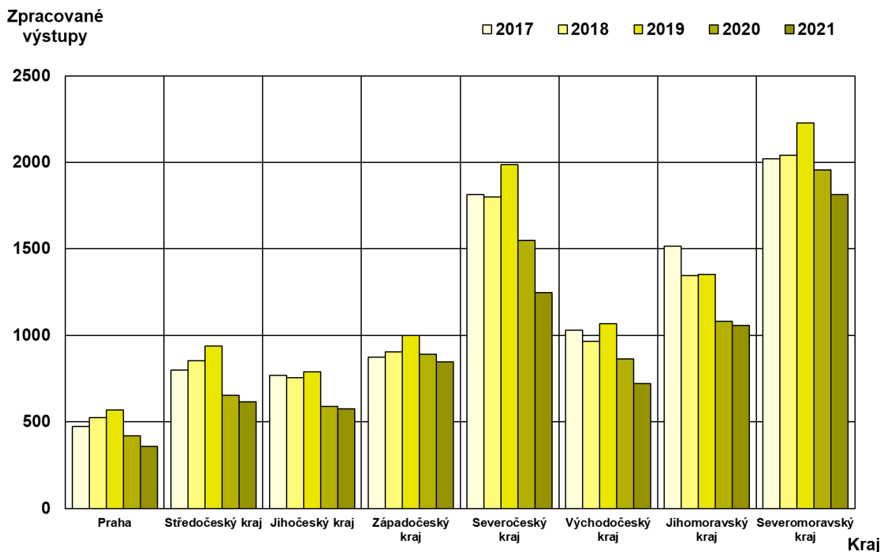
Graf 5 – Počet zpracovaných výstupů v rámci soudních krajů
