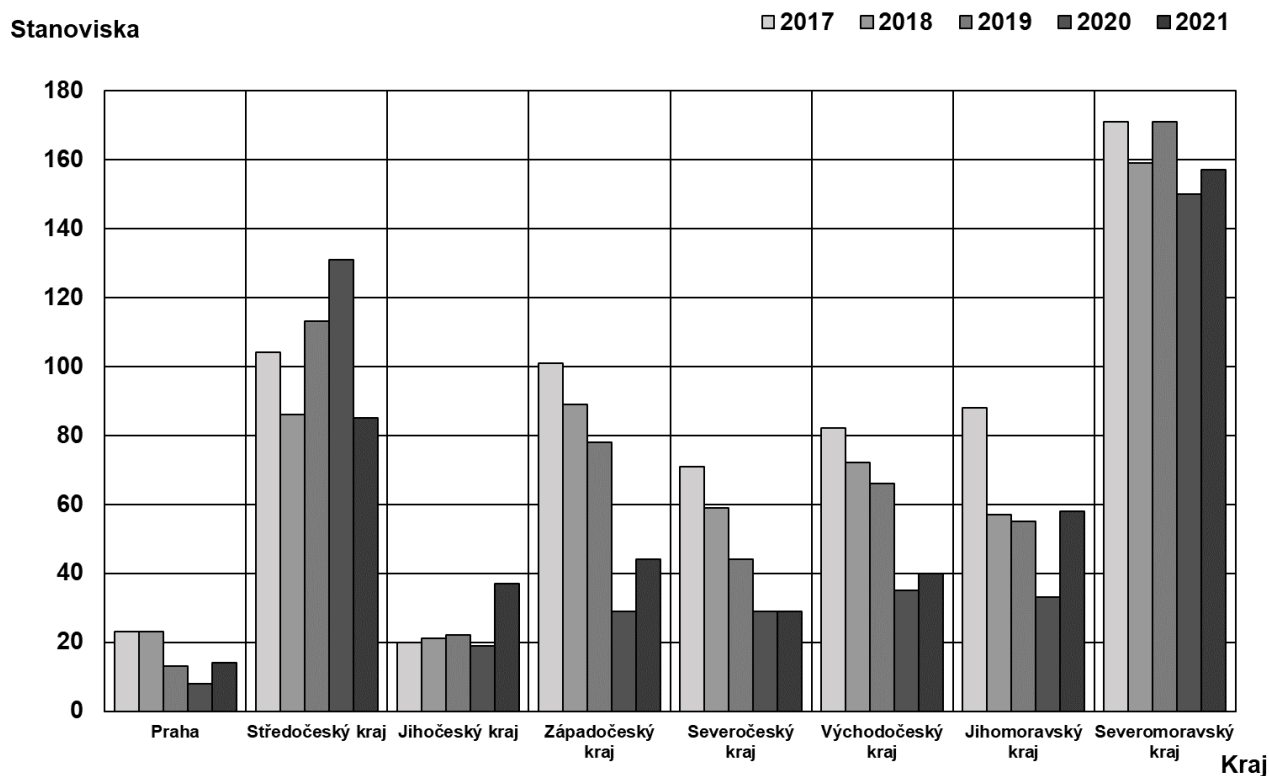
Graf 8 – Počet stanovisek k podmíněnému propuštění v rámci soudních krajů
