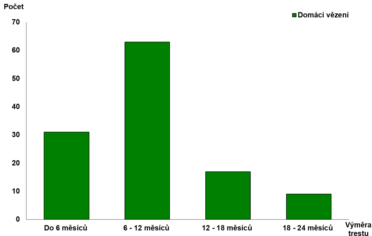
Graf 31 – Výměra trestu domácího vězení a povinnosti zdržet se ve stanoveném čase v obydlí v rámci podmíněného propuštění s dohledem za rok 2021
