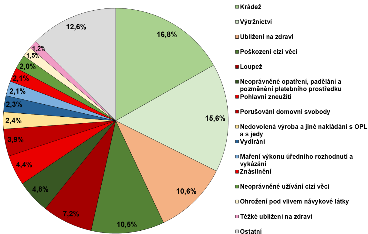
Graf 45 – Struktura provinění a protiprávních činů mládeže za rok 2021
