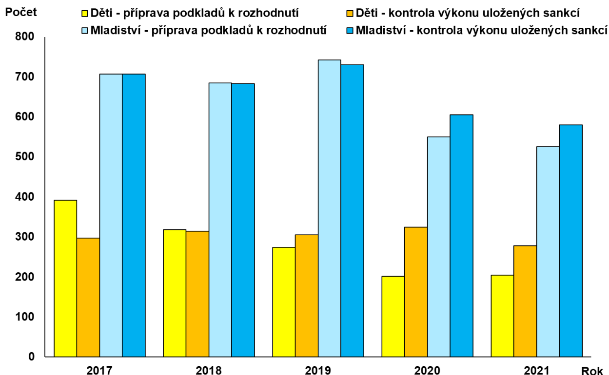
Graf 42 – Počet nových případů v agendě mládeže
