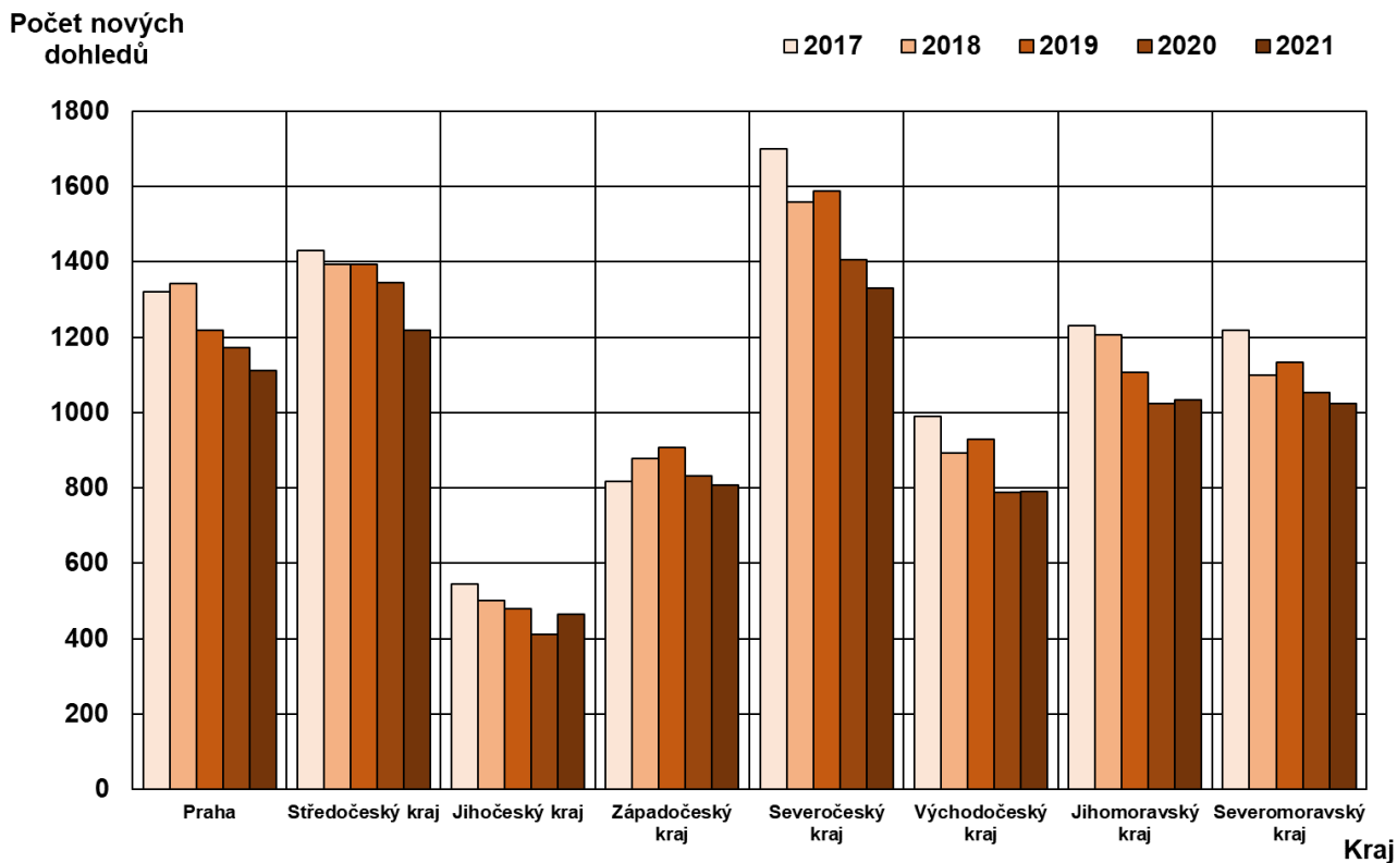
Graf 17 – Počet nových dohledů v rámci soudních krajů
