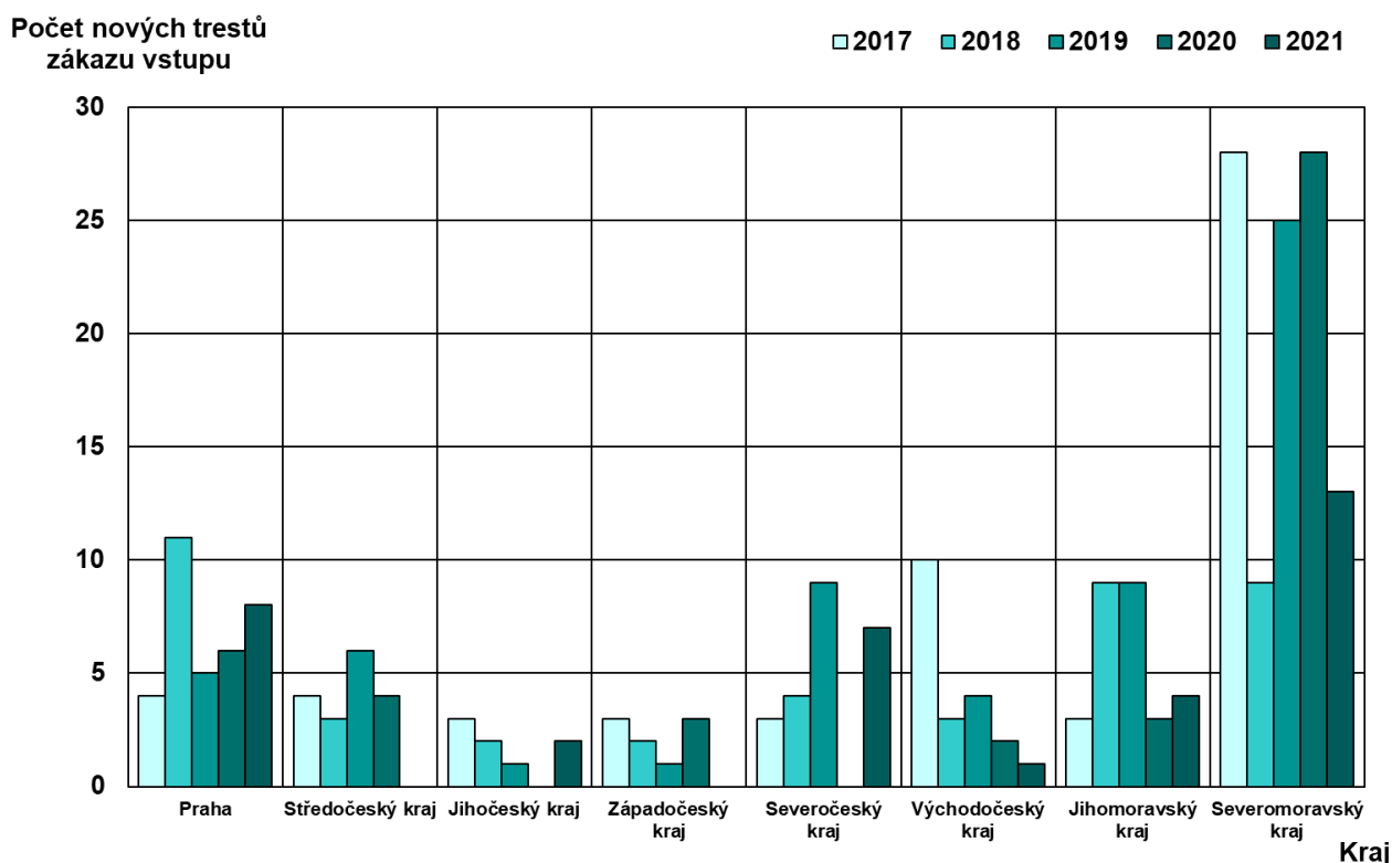
Graf 34 – Počet nových trestů zákazu vstupu v rámci soudních krajů
