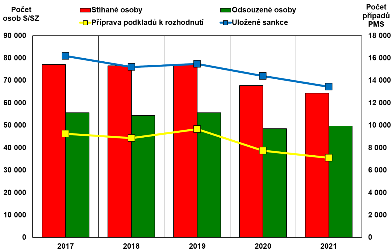
Graf 1 – Vývoj počtu stíhaných a odsouzených osob, počtu nových případů přípravy podkladů k rozhodnutí soudu či státního zastupitelství a uložených sankcí osobám 2017–2021
