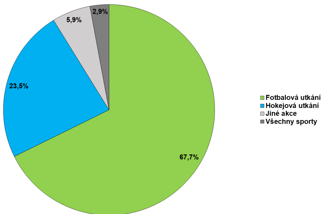
Graf 35 – Struktura věcné specifikace trestu zákazu vstupu v roce 2021
