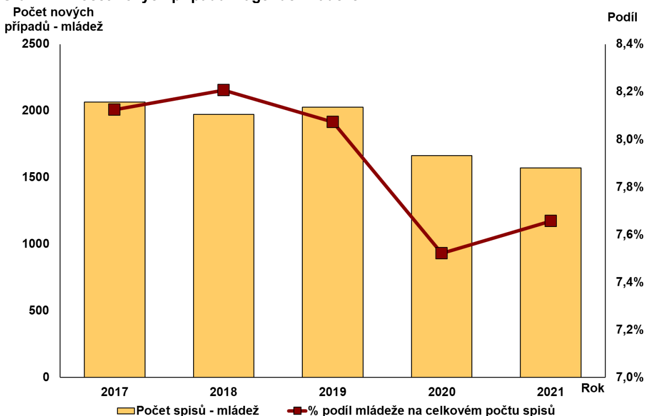
Graf 41 – Počet nových případů v agendě mládeže
