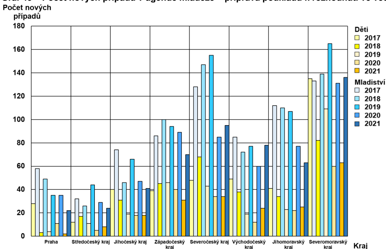
Graf 43 – Počet nových případů v agendě mládeže – příprava podkladů k rozhodnutí ve věci
