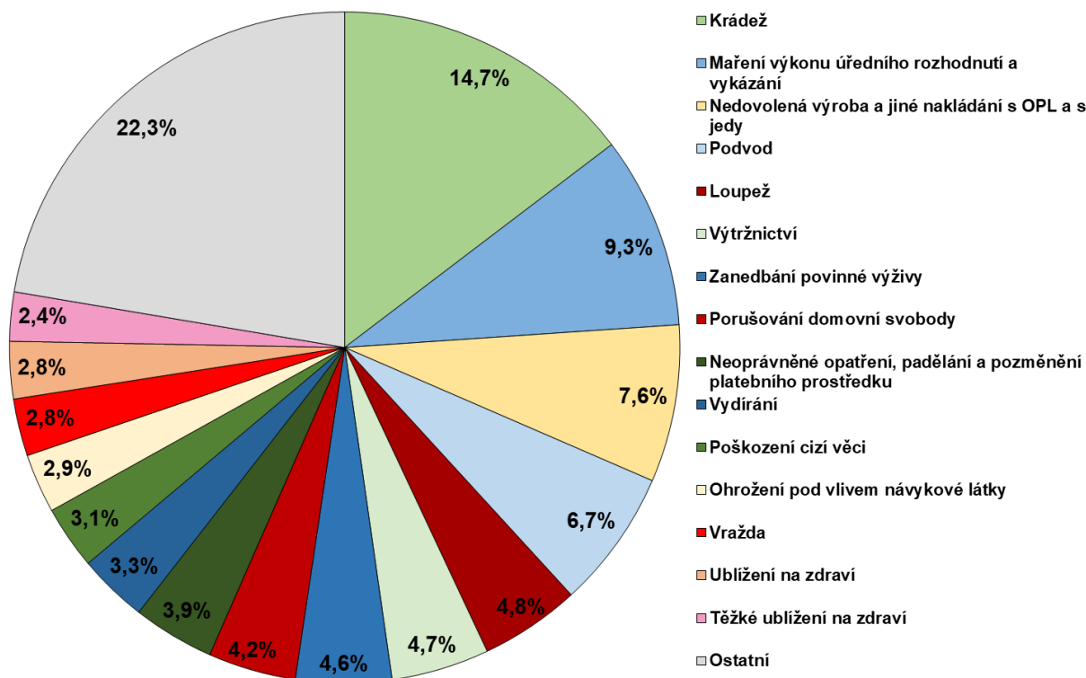
Graf 9 – Struktura trestné činnosti u stanovisek k podmíněnému propuštění za rok 2021
