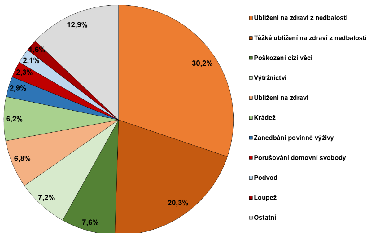
Graf 12 – Struktura případů, u kterých proběhla v roce 2021 mediace
