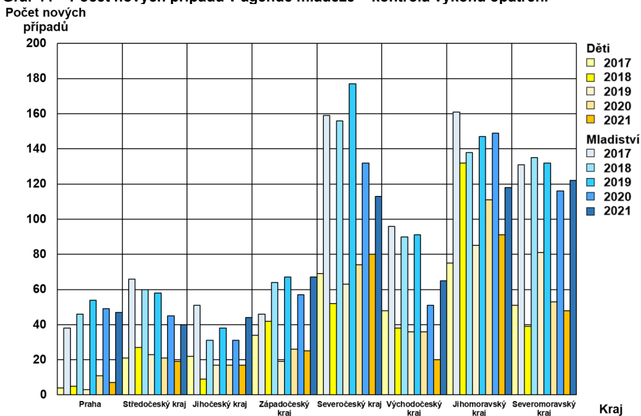
Graf 44 – Počet nových případů v agendě mládeže – kontrola výkonu opatření
