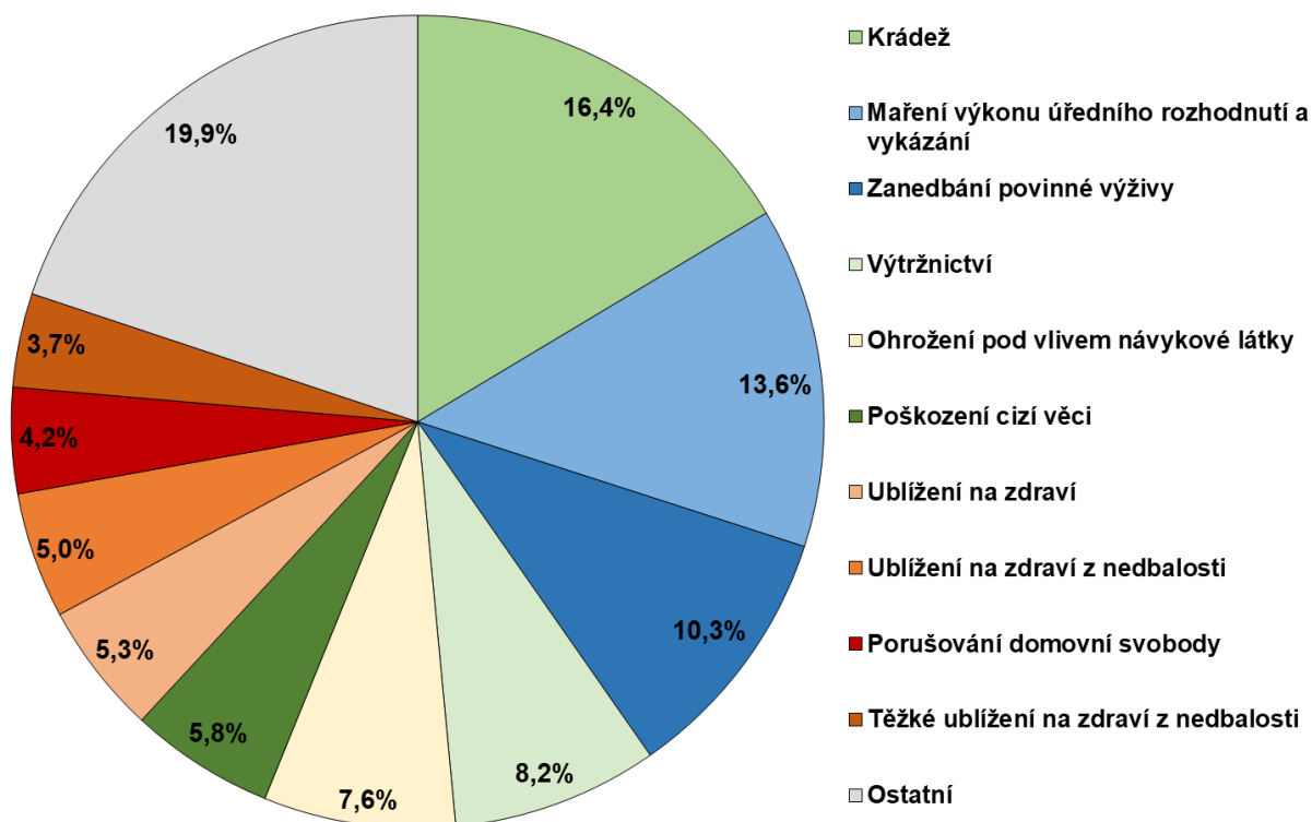
Graf 6 – Struktura trestné činnosti u zprostředkování řešení konfliktu za rok 2021
