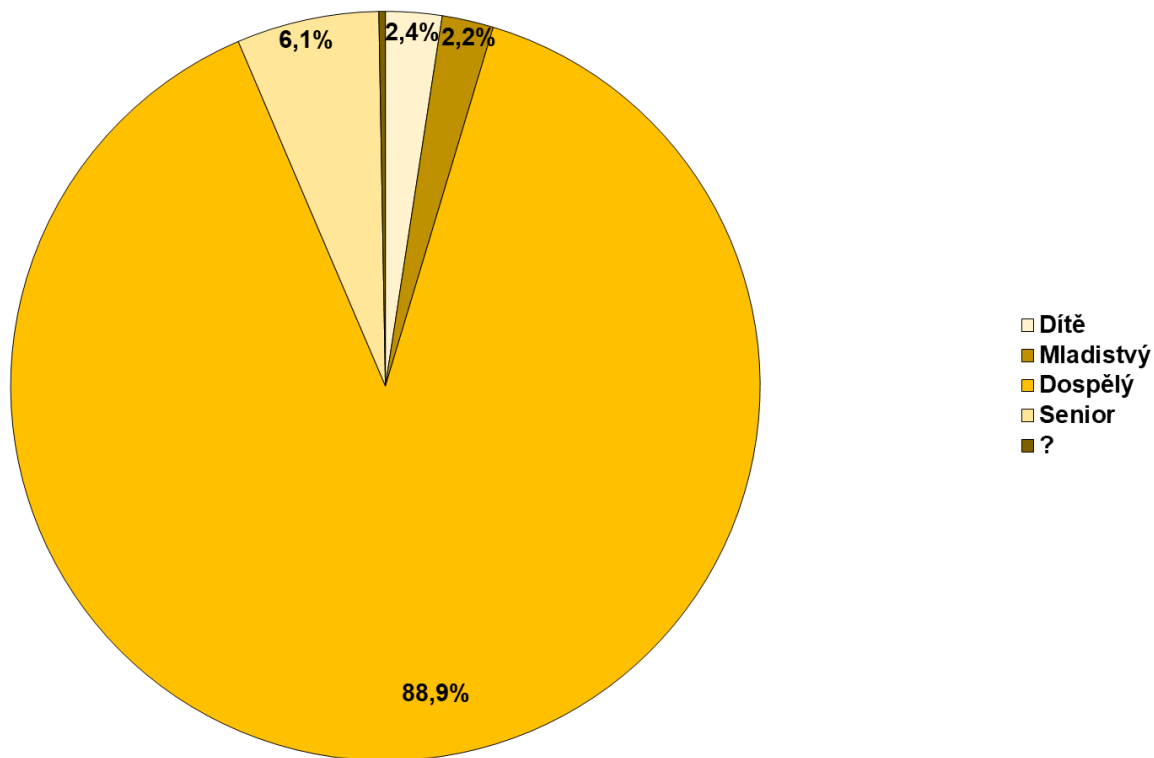
Graf 15 – Struktura obětí trestných činů dle věku v roce 2021
