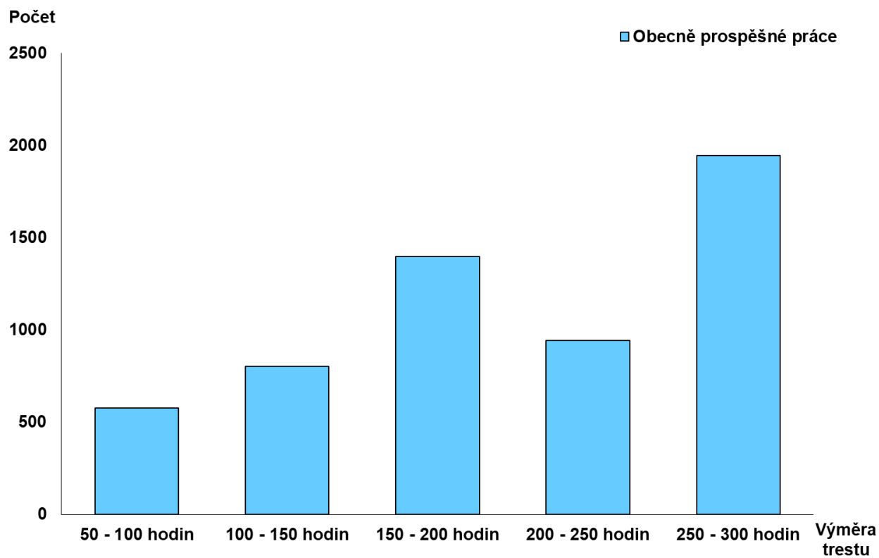
Graf 26 – Výměra trestu obecně prospěšných prací za rok 2021
