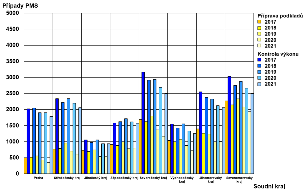
Graf 3 – Vývoj počtu nových případů přípravy podkladů k rozhodnutí soudu či státního zastupitelství a uložených sankcí osobám v soudních krajích 2017–2021
