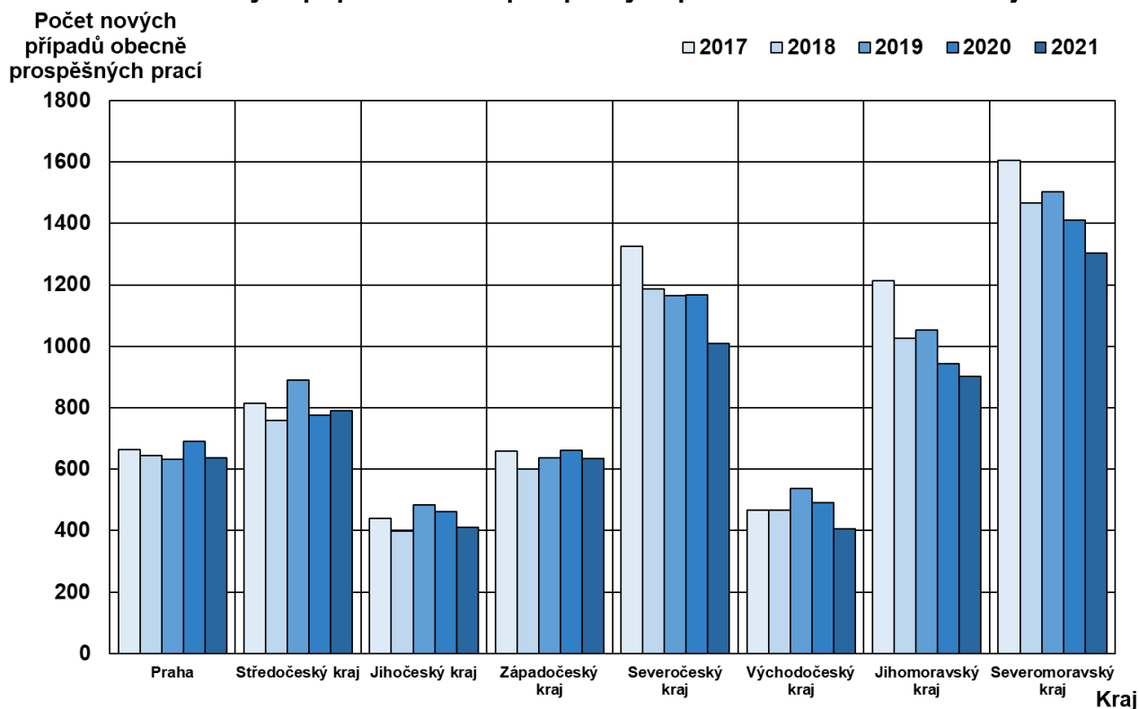
Graf 24 – Počet nových případů obecně prospěšných prací v rámci soudních krajů
